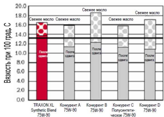
Сравнительный анализ вязкостей свежего масла и после испытания на сдвиг KRL при 1000С, GL-5 75W-90
